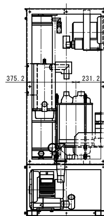
A-A section view A-A断面
